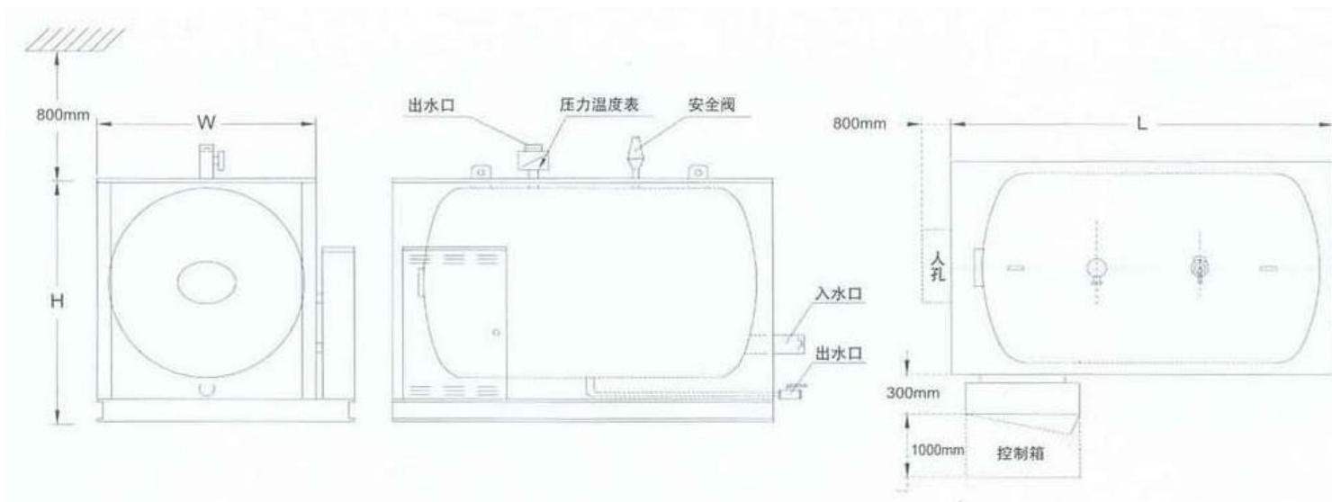
EHWC 卧式型号尺寸
