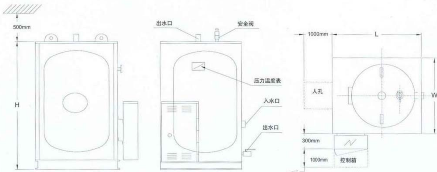
EHWC 立式型号尺寸
